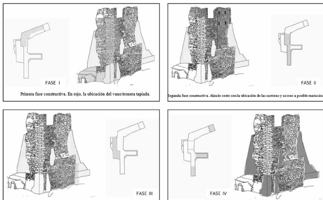
Fig. 6. Fases constructivas de la Torre del Homenaje.
