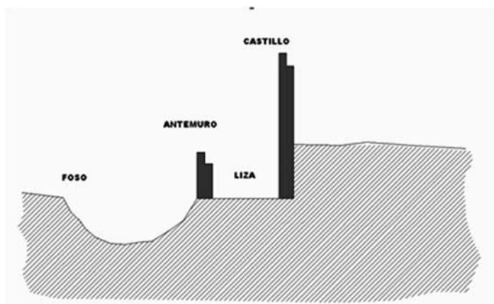
Figura 10. Esquema común de foso con falsabraga.
