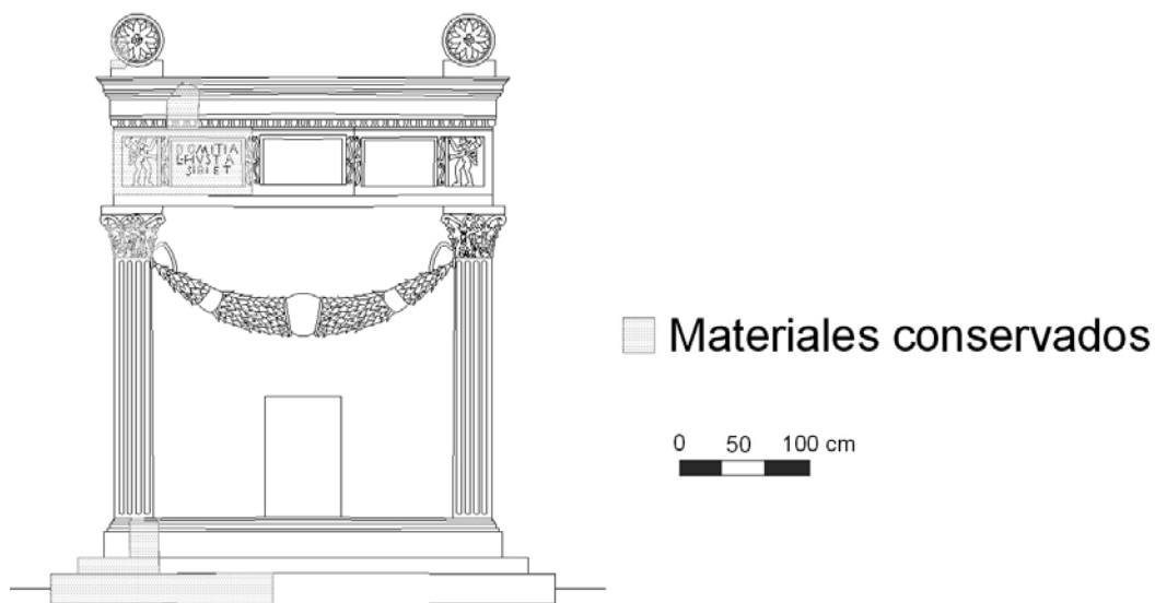
Figura 6. Reconstrucción volumétrica hipotética del monumento funerario de “La Calerilla” de Hortunas de Requena (Valencia).
