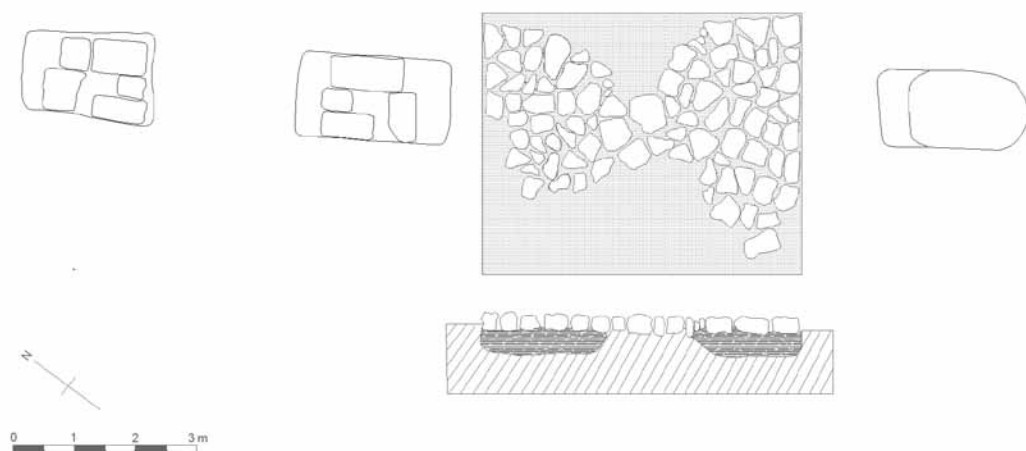
Figura 4. Figura 4. Planimetría de la parte central de la necrópolis de “La Calerilla” de Hortunas.
