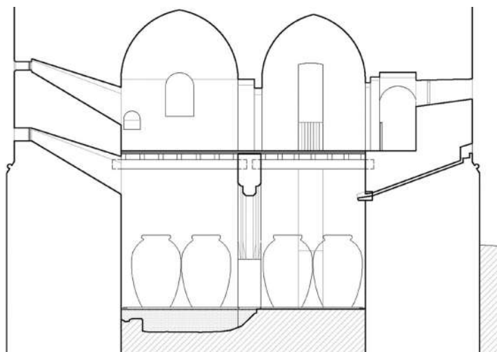
Sección del torreón según hipótesis de F. Blay sobre sección del proyecto. En: BALAGUER DEZCALLAR, M a Josefa; BLAY GARCÍA, Francisco y MARTÍNEZ VALLE, Asunción. “Proceso de investigación y restauración de elementos del sistema defensivo de Requena con testimonios de la actividad vitícola”. En: Paisajes y patrimonio cultural del vino y otras bebidas psicotrópicas. Requena, Valencia, España, del 12 al 15 de abril de 2011. Requena, Ayuntamiento, 2013, 391-396.
