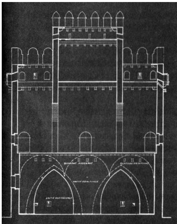
Sección de la torre del Canyamel (Llevant, Mallorca)
