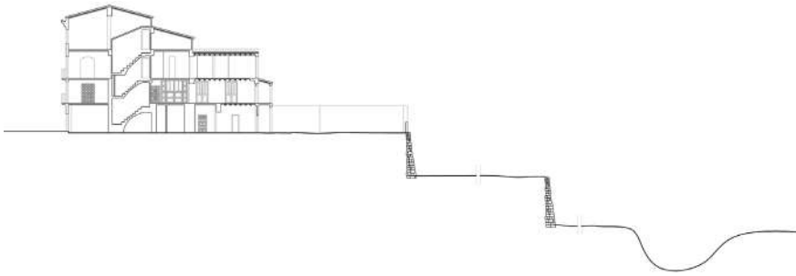
Casa del retablo | Sección longitudinal |
