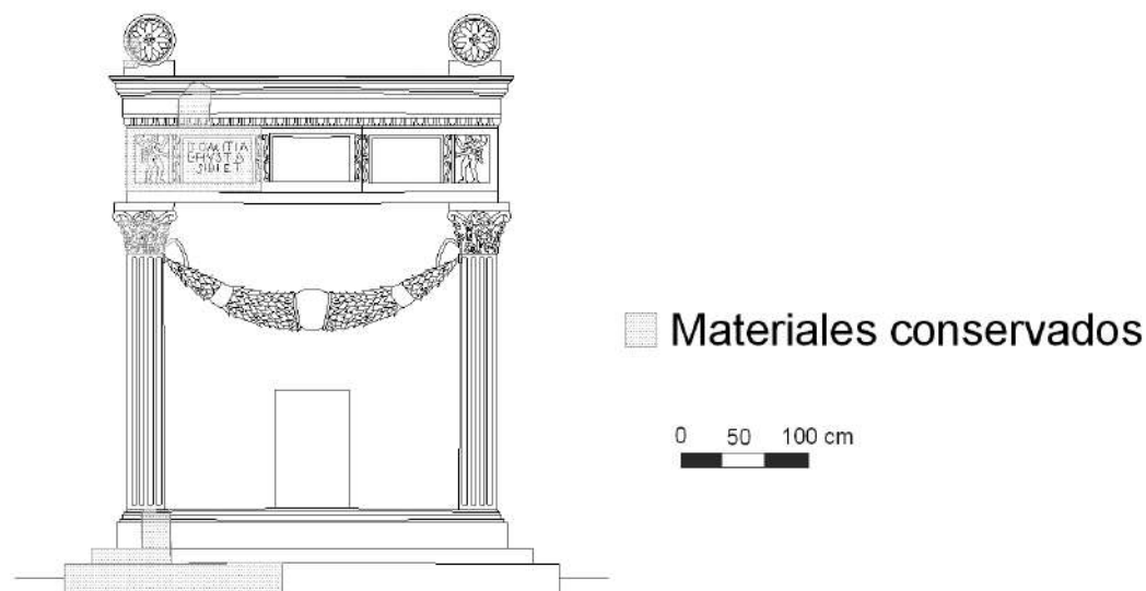
Figura 3. Alzado del monumento funerario de Domitia Iusta a partir de los materiales conservados
