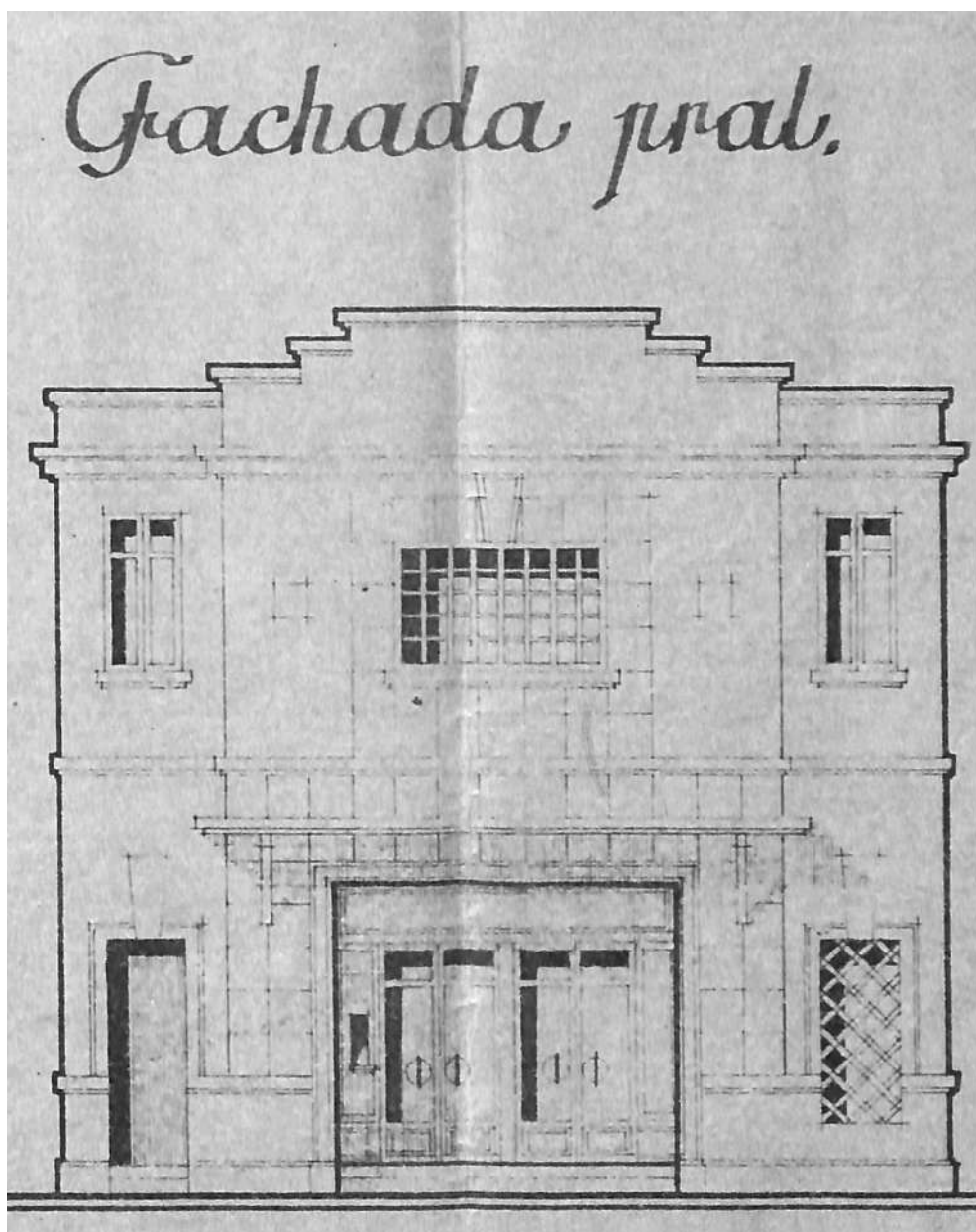
1952, enero, 5 – 1954, septiembre, 27. Requena. Plano de la fachada del cinematógrafo de Casas de Eufemia promovido por Ricardo García Soldevilla (AMRQ 2.076/113).
